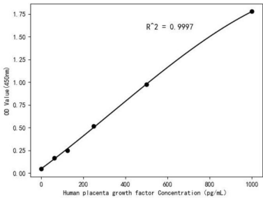
Figure1. 96 孔板分析的 Human PLGF 标准曲线。数据和曲线仅供参考，实验者需根据自己的实验建立标准曲线
